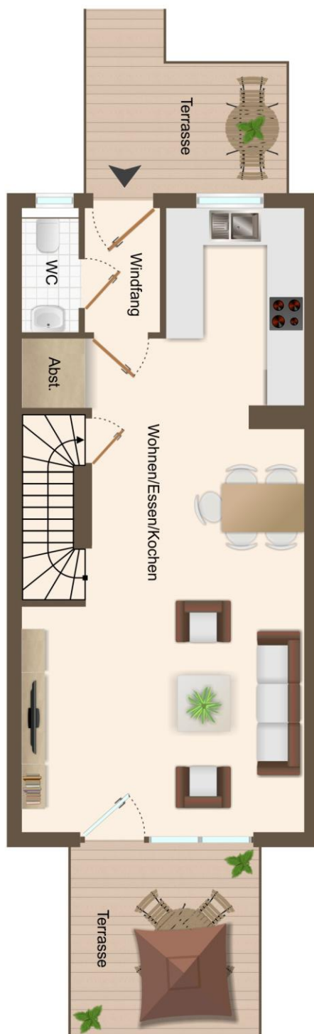
Grundriss Erdgeschoss WE4
